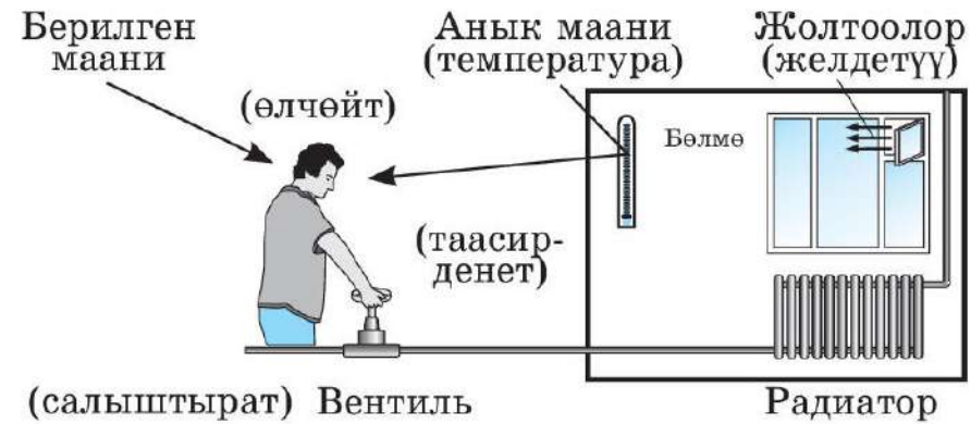
47-сүрөт. Бөлмөдө абанын температура-сын жөнгө салуунун принциби.
